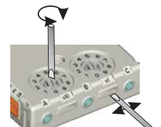
FIGURA 2: SELECTORES DE DIRECCIÓN GIRATORIOS Y DECÁDICOS
