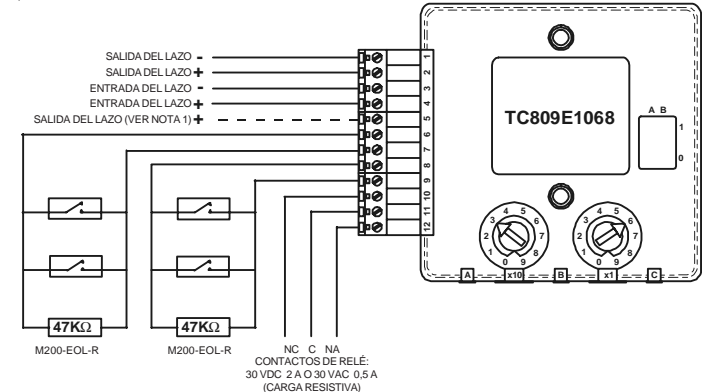
FIGURA 4: CONEXIONES DEL MÓDULO DE ENTRADA DOBLE Y SALIDA ÚNICA TC809E1068
