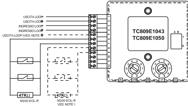
FIGURA 3: CABLAGGIO DEL MODULO A INGRESSO SINGOLO TC809E1043 E A INGRESSO DOPPIO TC809E1050
