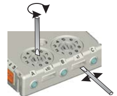
FIGURA 2: SWITCH ROTATIVI PER INDIRIZZAMENTO DECIMALE
