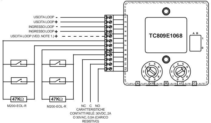
FIGURA 4: CABLAGGIO DEL MODULO A USCITA SINGOLA E DOPPIO INGRESSO TC809E1068
