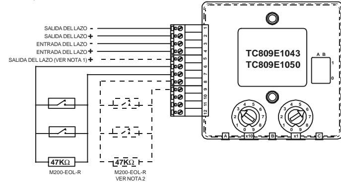
FIGURE 3: CONEXIONES DE LOS MÓDULOS TC809E1043 DE ENTRADA ÚNICA Y TC809E1050 DE ENTRADA DOBLE
